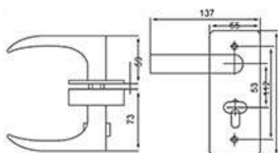
ELHL-102 Double Door
