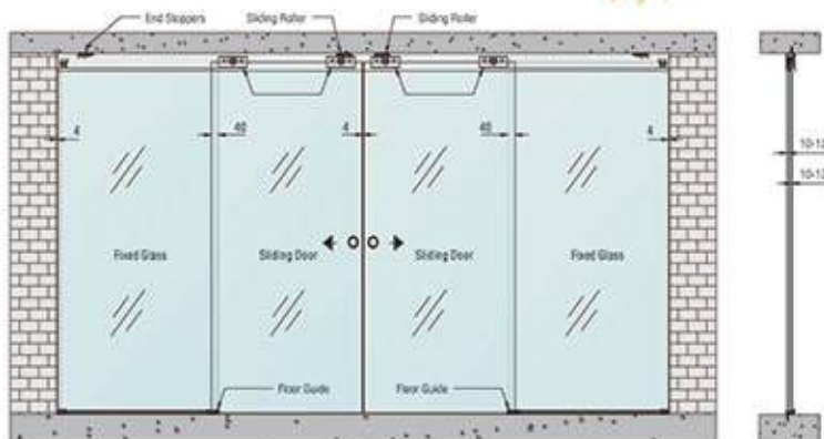
Double door structure
