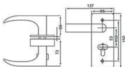
ELHL-101 Single Door
