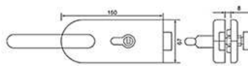
ELHL-012 Double Door
