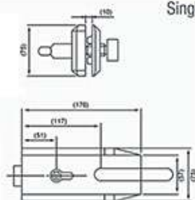
ELHL-001 Single Door
