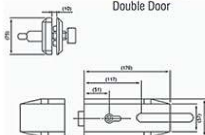
ELHL-002 Double Door
