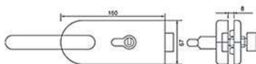
ELHL-011 Single Door
