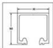
Track Dimension :
